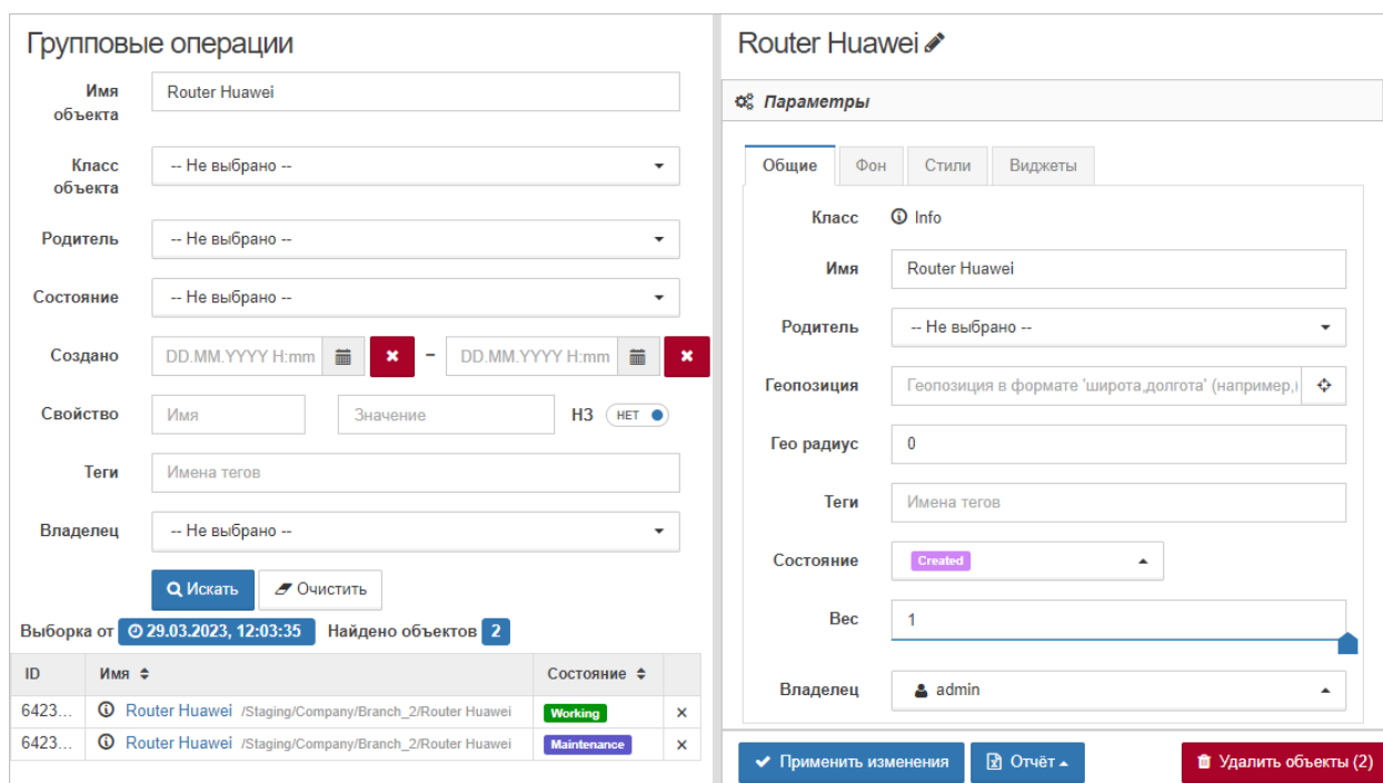
Рис. 108. Настройка найденных объектов
