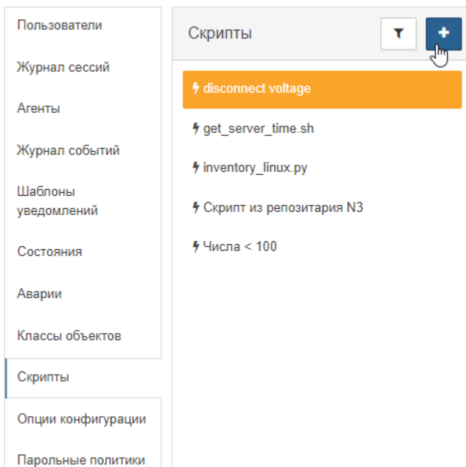
Рис. 134. Репозиторий скриптов
