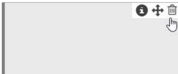
Рис. 30. Удаление подложки
