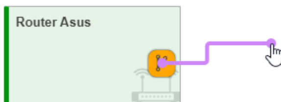
Рис. 7. Создание связи
