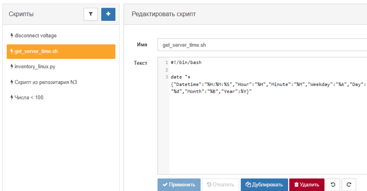
Рис. 135. Редактирование скриптов
