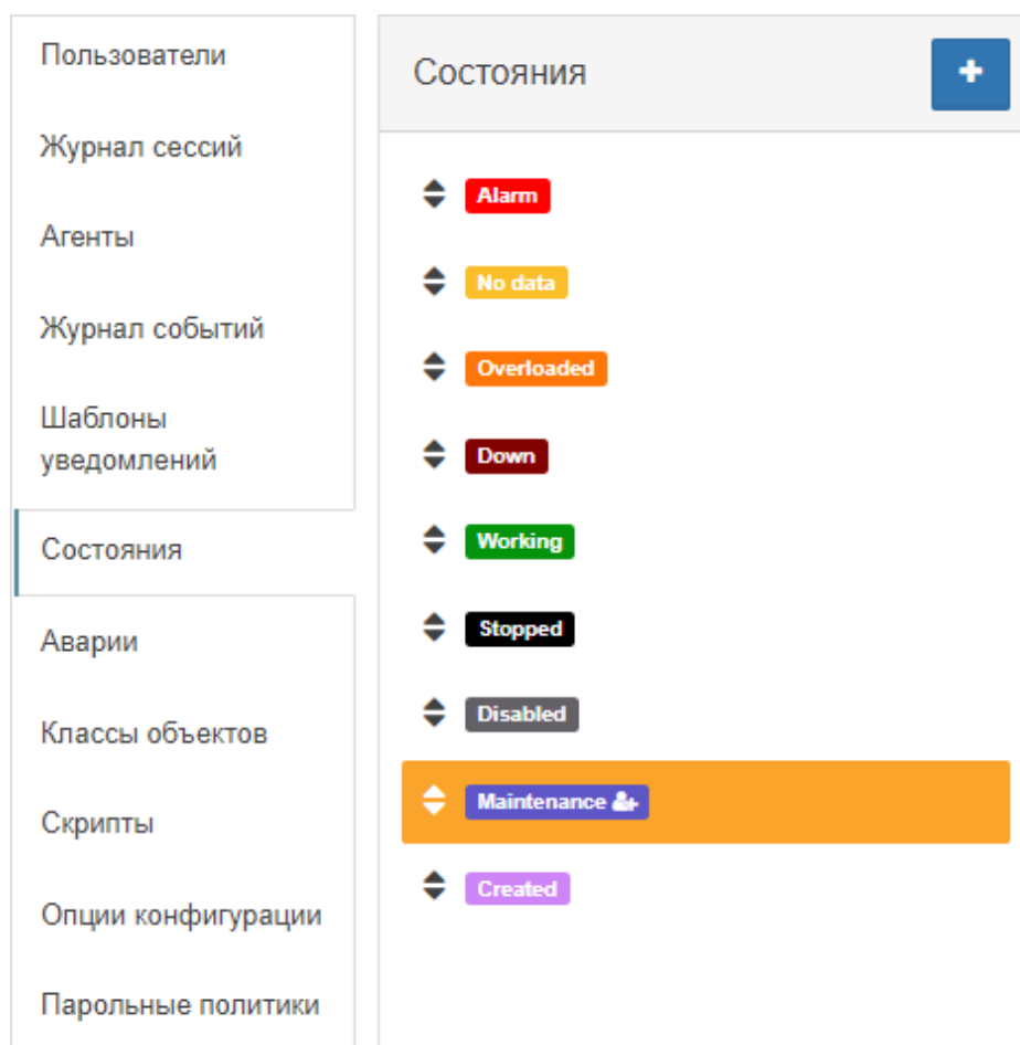
Рис. 127. Список состояний
