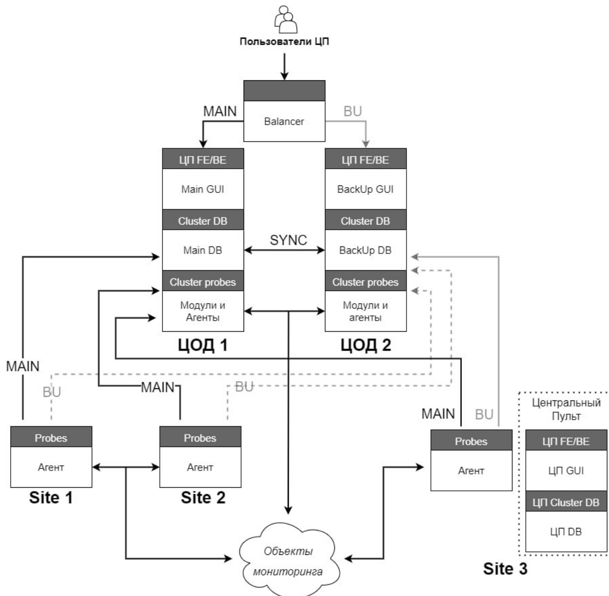
Рис. 2. Отказоустойчивое исполнение системы
