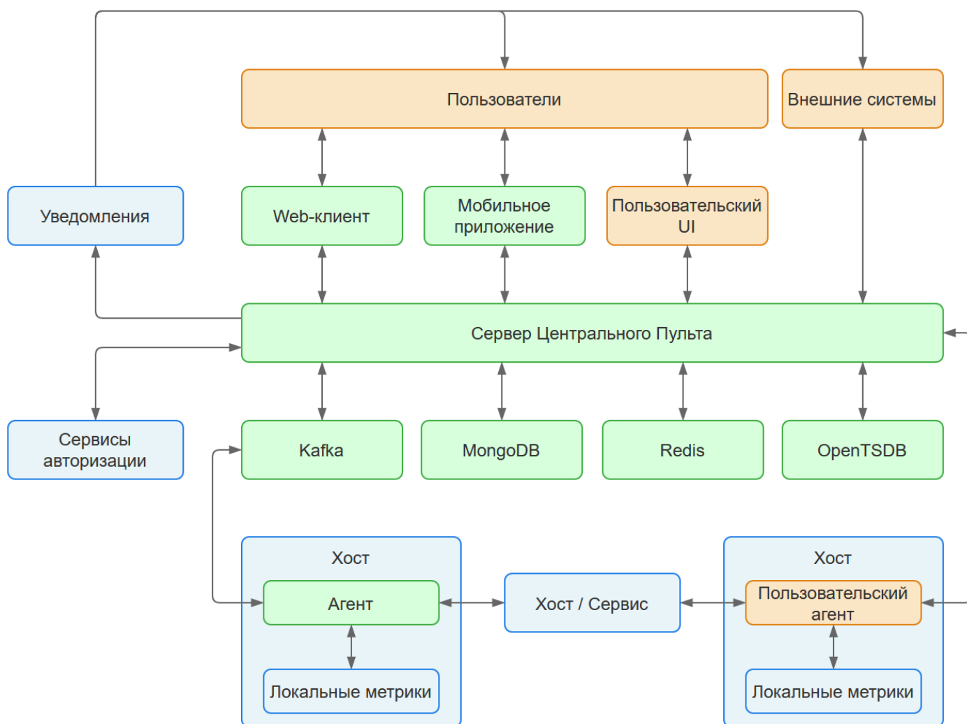
Рис. 1. Архитектура платформы "Центральный Пульт"
