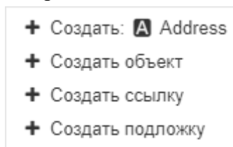
Рис. 12. Контекстное меню
