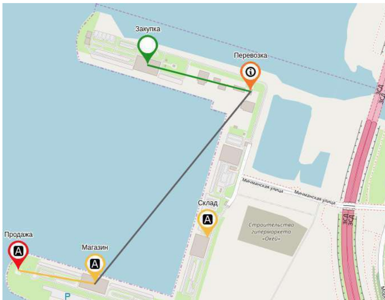
Рис. 5. Геокарта
