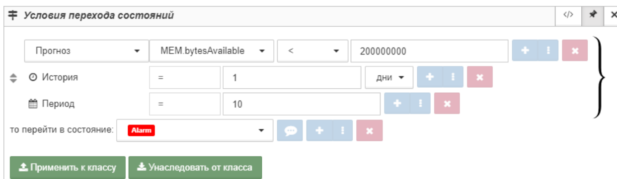
Рис. 88. Пример правила для прогнозирования значения метрики
