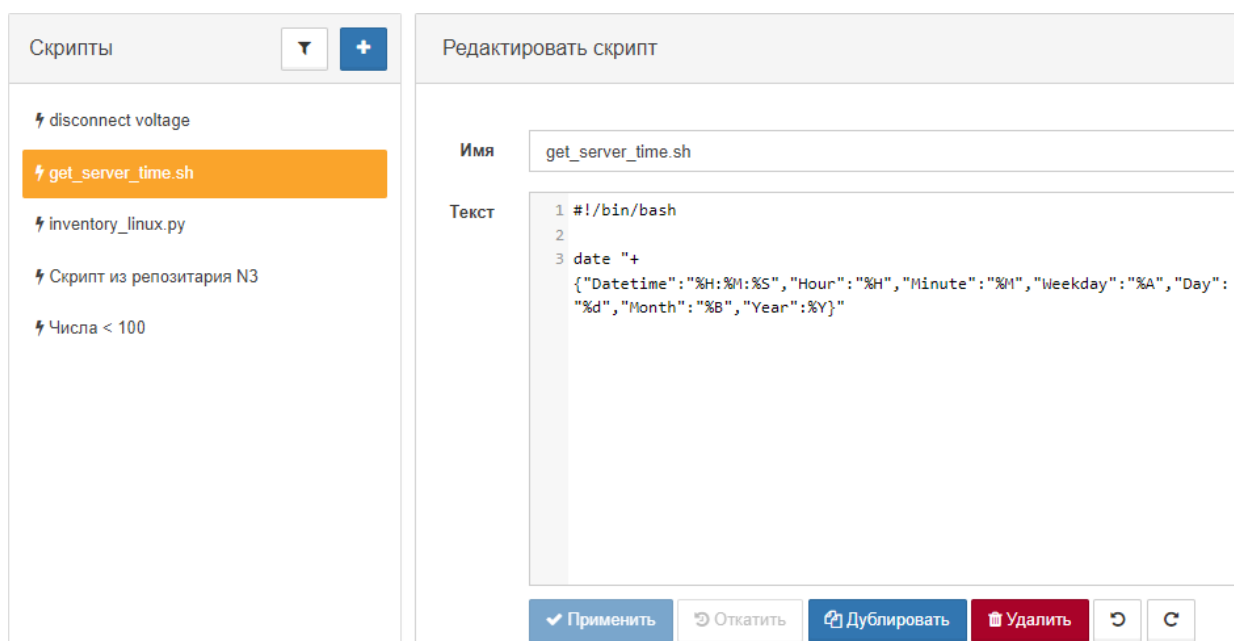
Рис. 135. Редактирование скриптов
