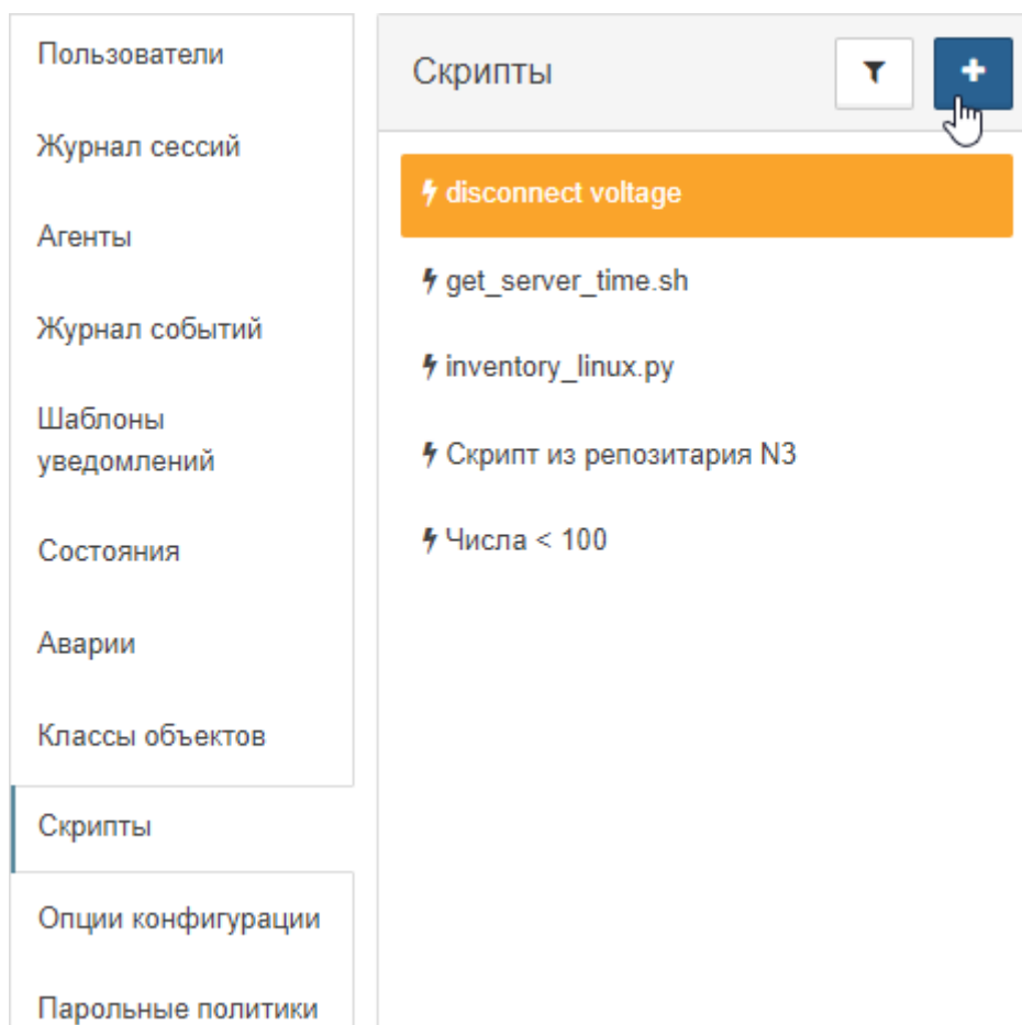
Рис. 134. Репозитарий скриптов
