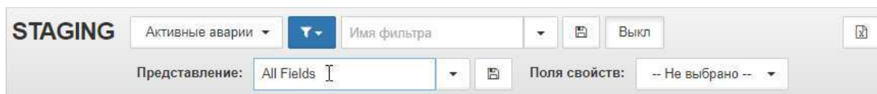
Рис. 68. Сохранение представления
