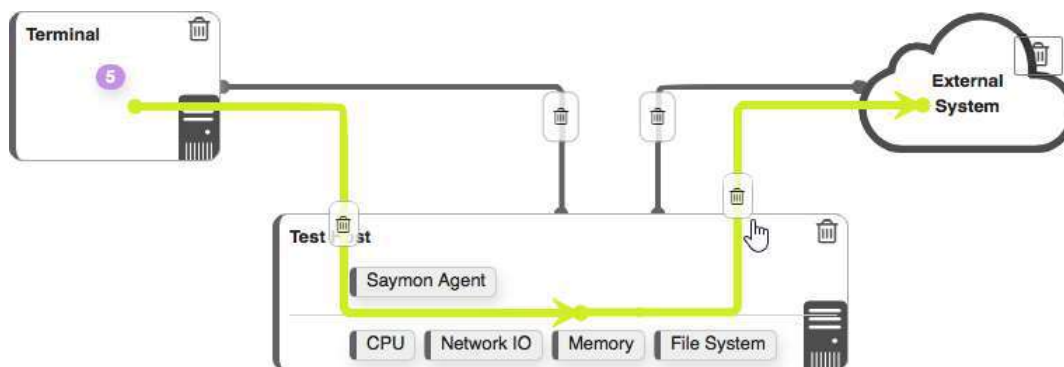
Рис. 25. Удаление потока
