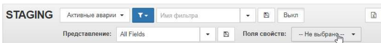
Рис. 69. Поля свойств
