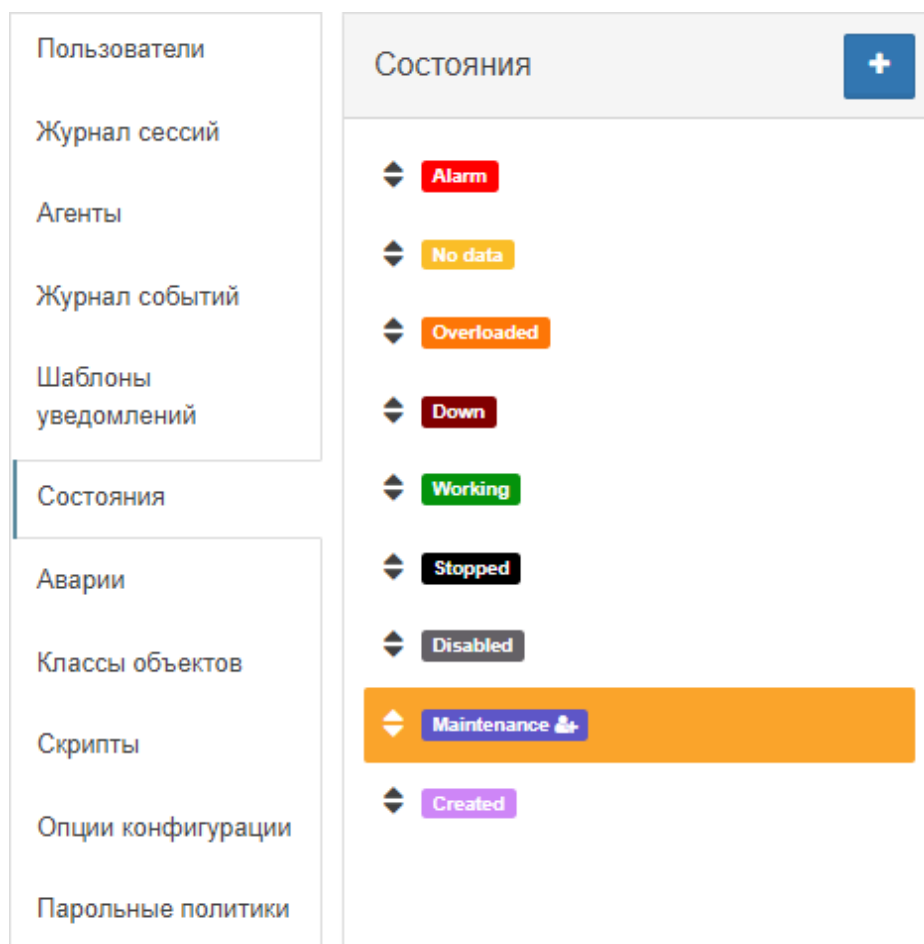
Рис. 127. Список состояний
