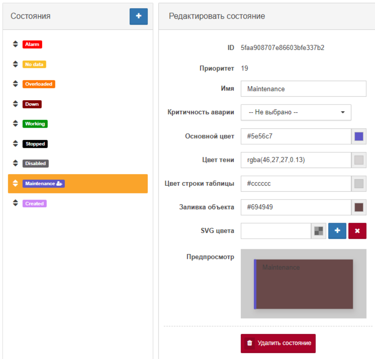
Рис. 128. Редактирование состояния
