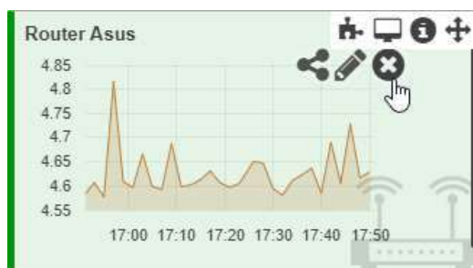
Рис. 90. Удаление виджета
