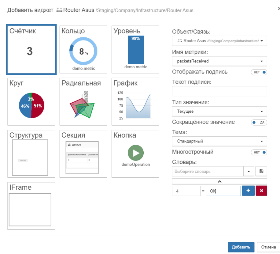
Рис. 92. Добавление виджета "Счётчик"
