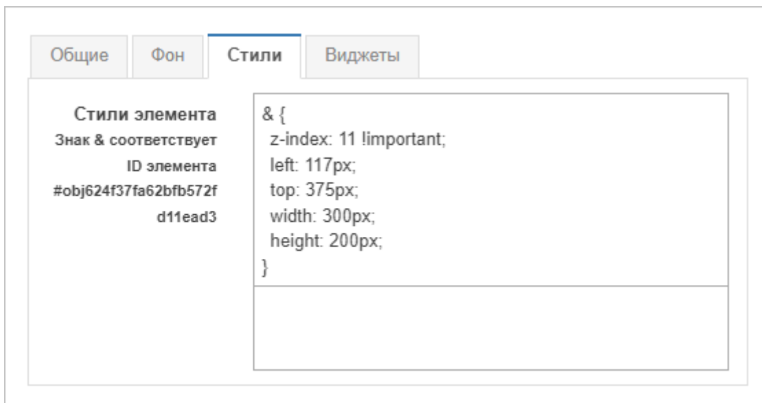
Рис. 6. Вкладка "Стили" объекта с фиксированным z-индексом
