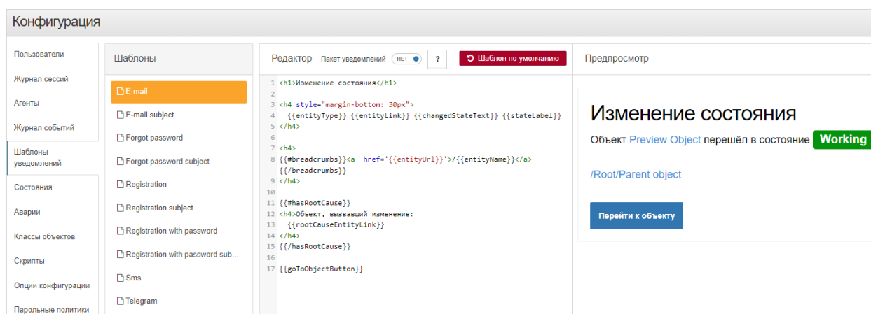
Рис. 126. Настройка шаблонов уведомлений
