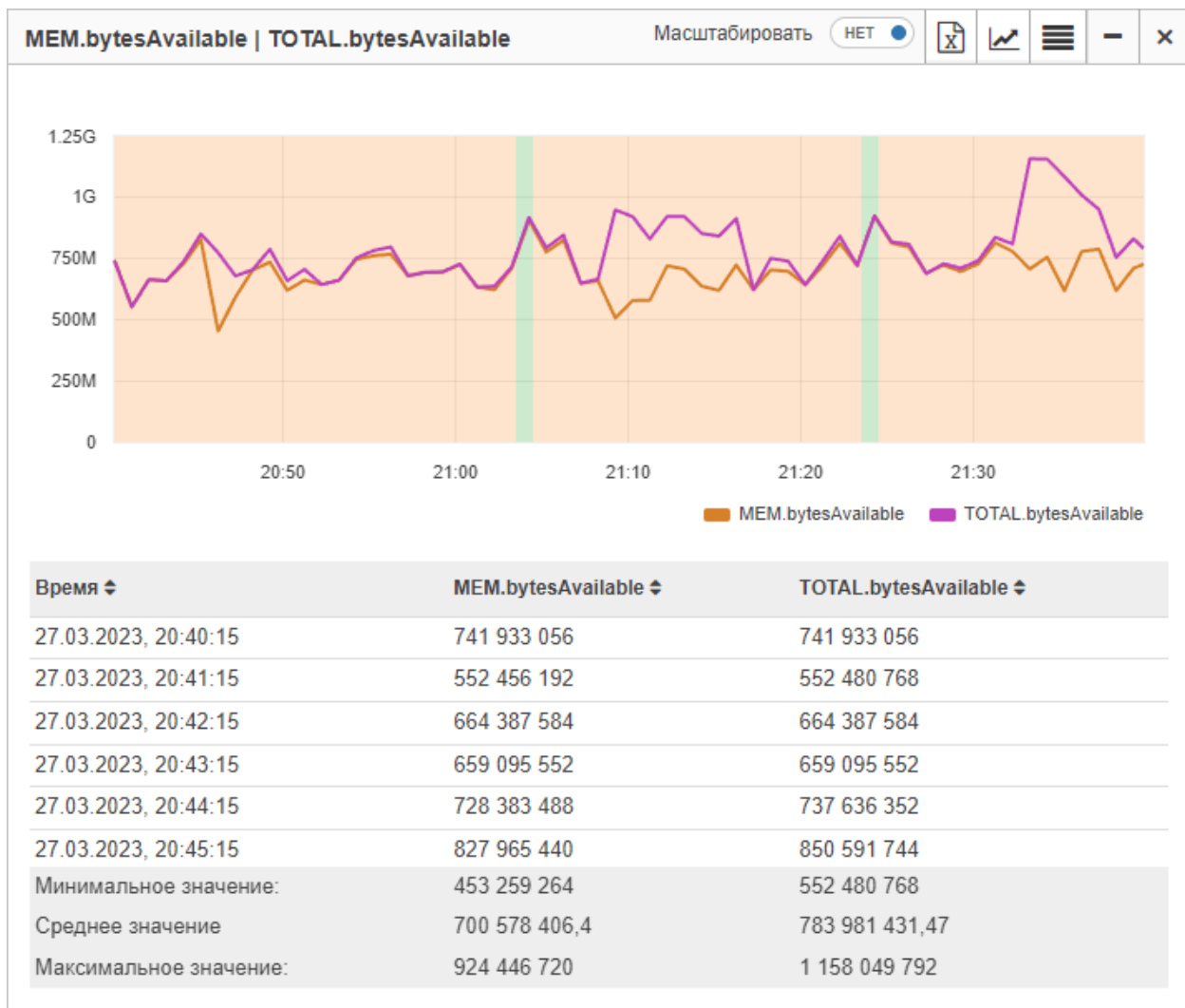
Рис. 100. Пример мультиграфика
