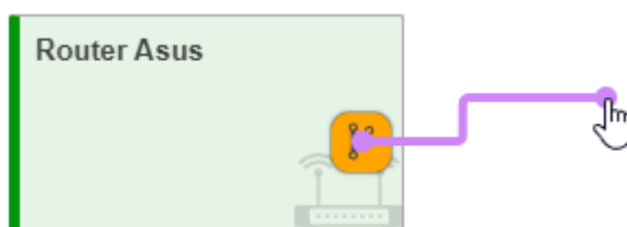
Рис. 7. Создание связи
