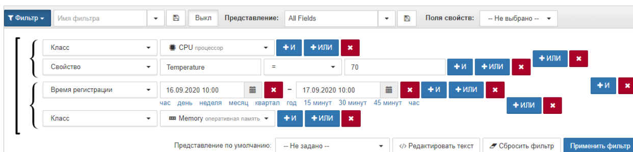
Рис. 73. Фильтр аварий
