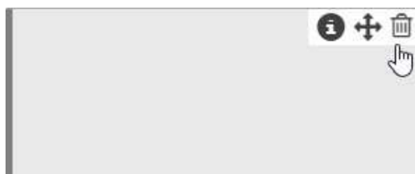
Рис. 30. Удаление подложки
