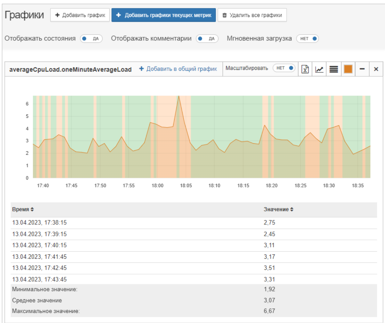
Рис. 97. Пример графика
