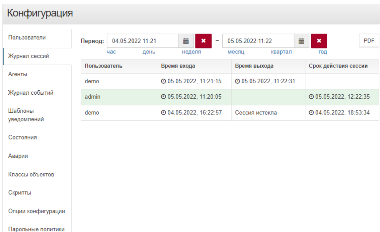
Рис. 124. Журнал сессий
