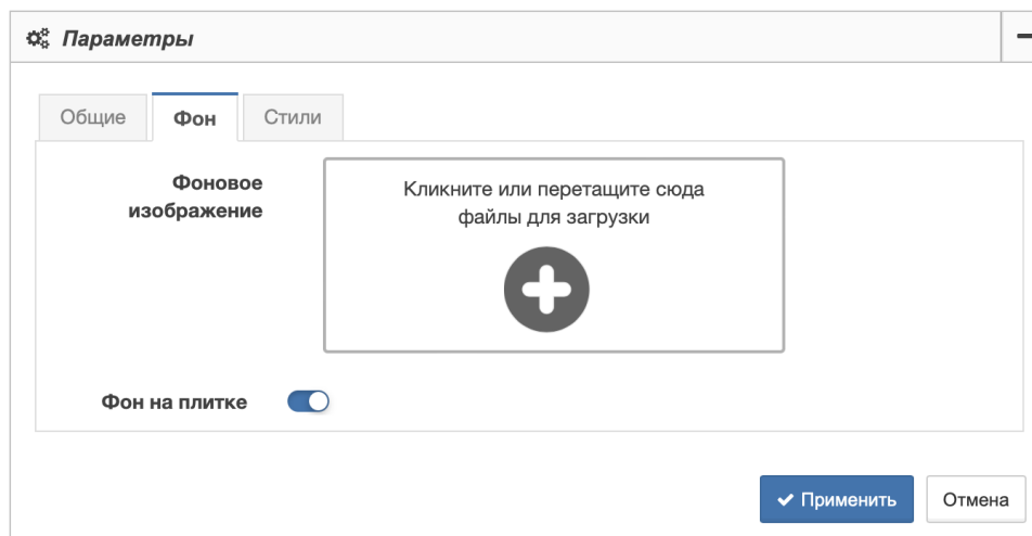
Рис. 28. Фон подложки
