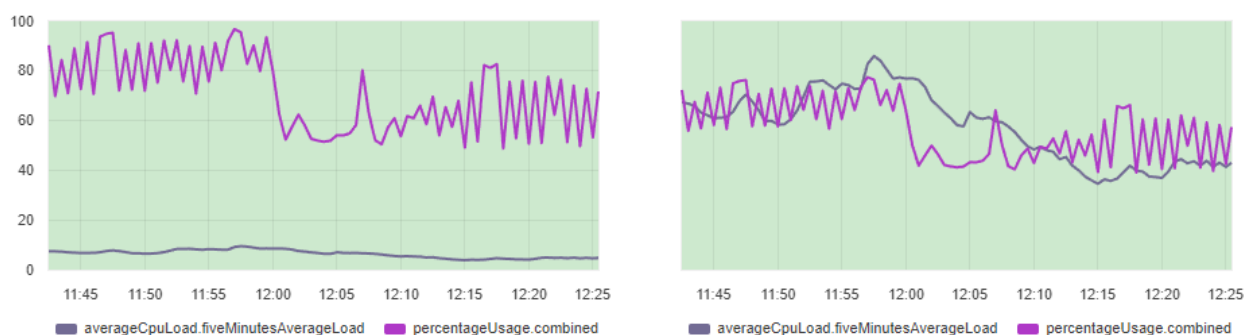
Рис. 101. Масштабирование значений на мультиграфике
