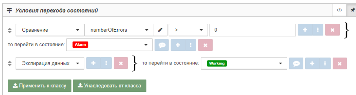
Рис. 61. Пример настройки условия с типом "Экспирация данных"
