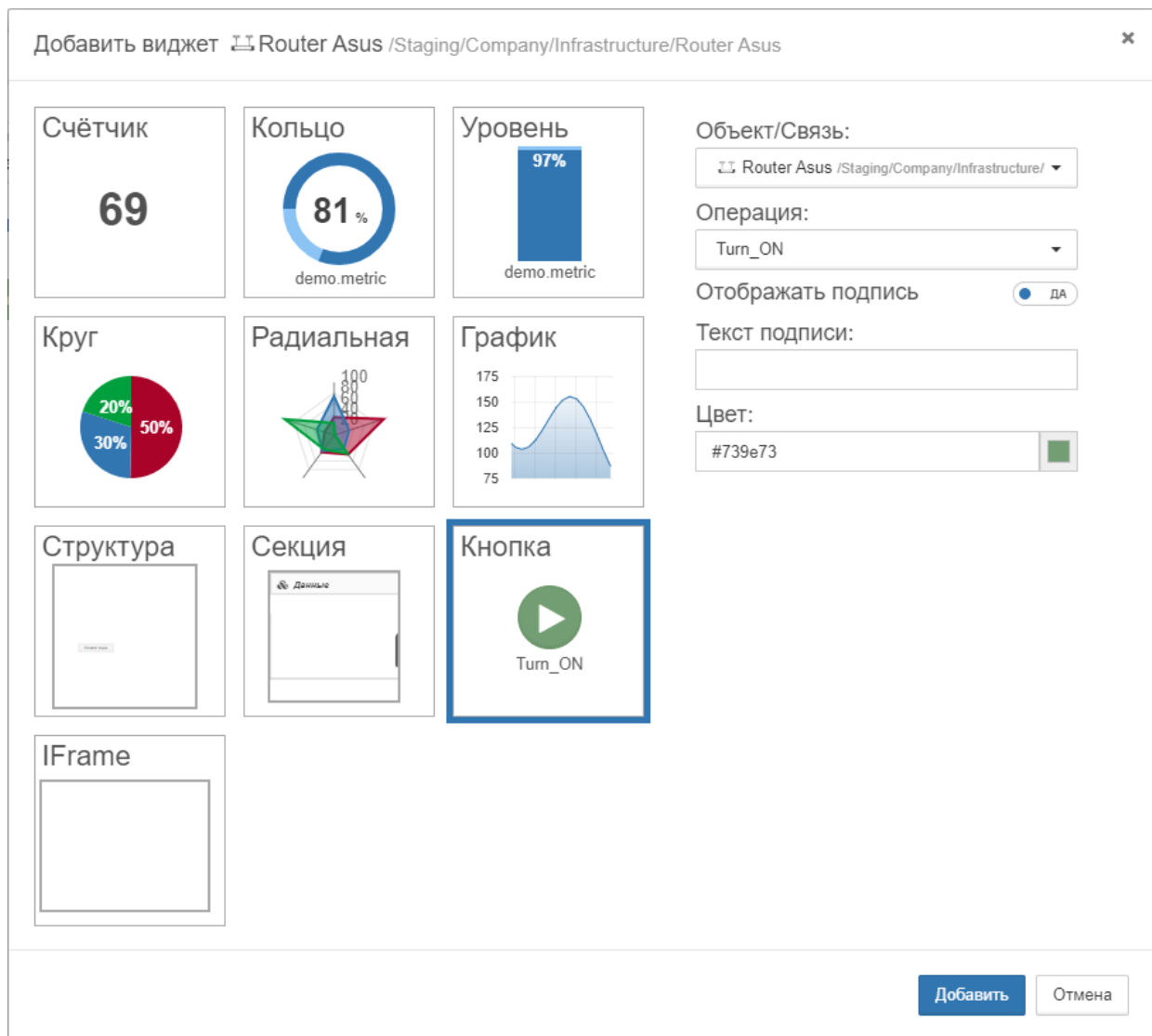
Рис. 84. Добавление виджета "Кнопка"
