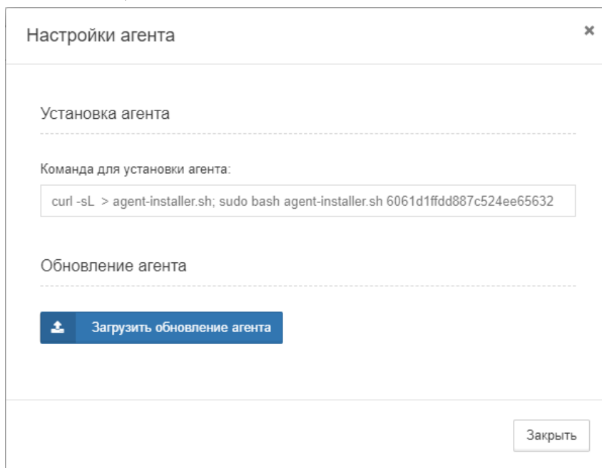
Рис. 3.1.1.1.2. Команда для установки агента
