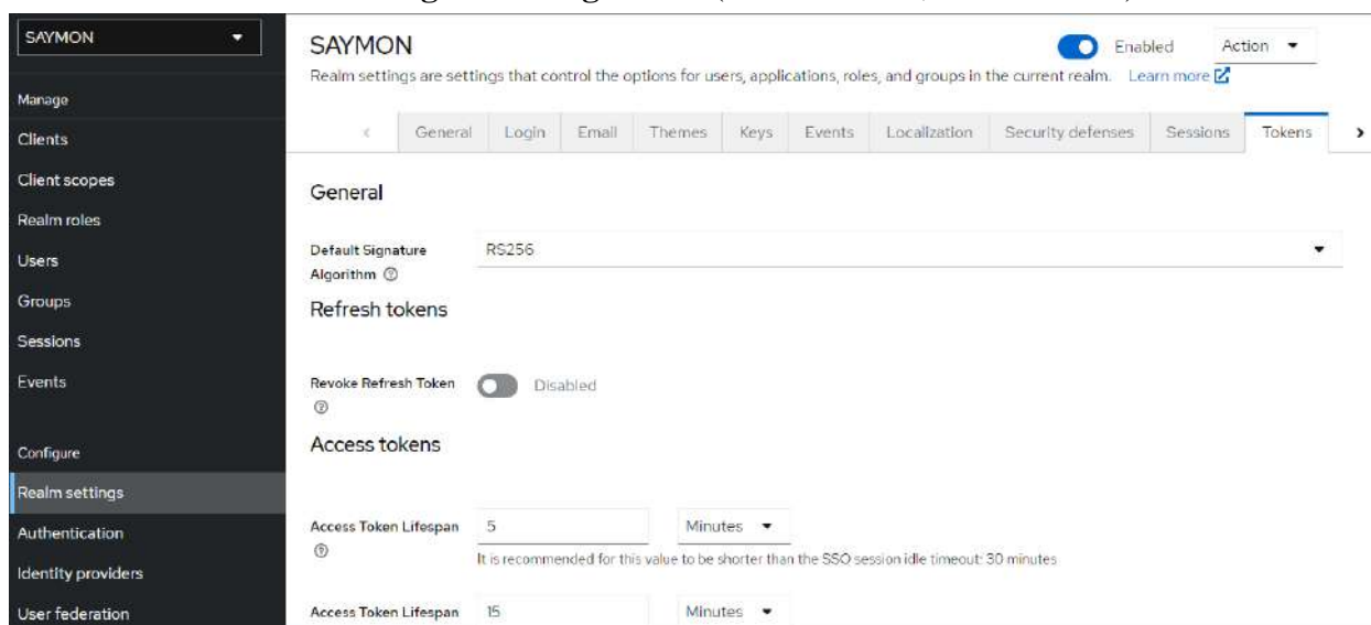
Рис. 3.5.3.1.2. Проверка алгоритма подписи токенов
