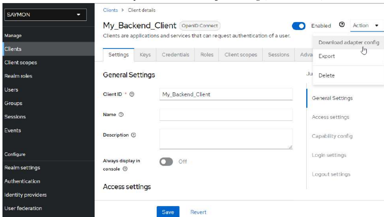
Рис. 3.5.3.1.8. Получение файла конфигурации Backend-клиента
