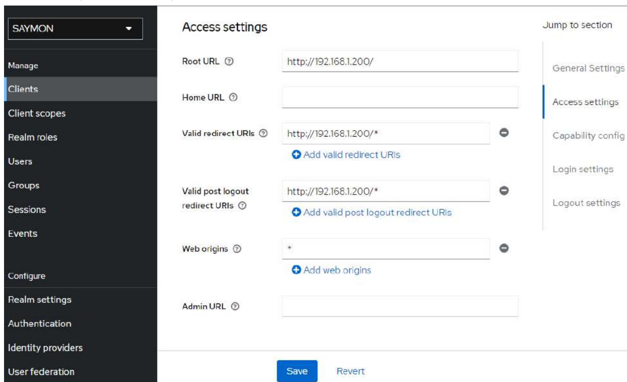
Рис. 3.5.3.2.3. Отключение клиентской аутентификации
