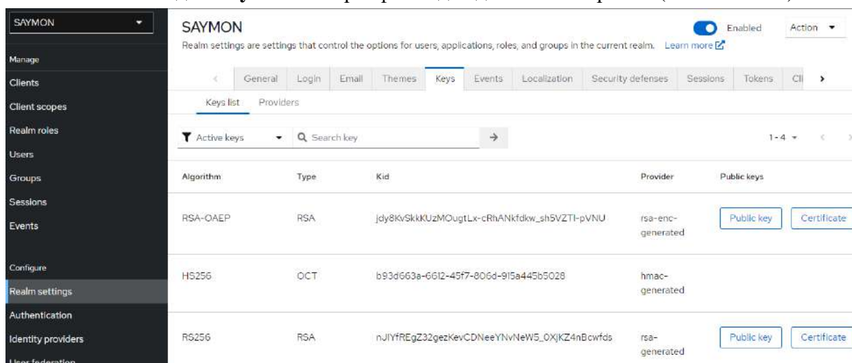
Рис. 3.5.3.1.3. Получение сертификата
