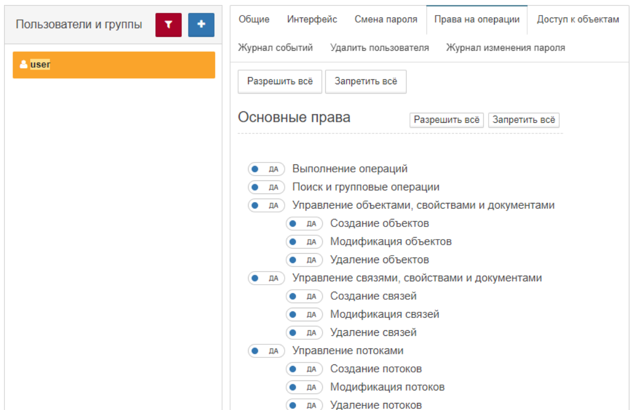
Рис. 3.7.4.1. Права на операции
