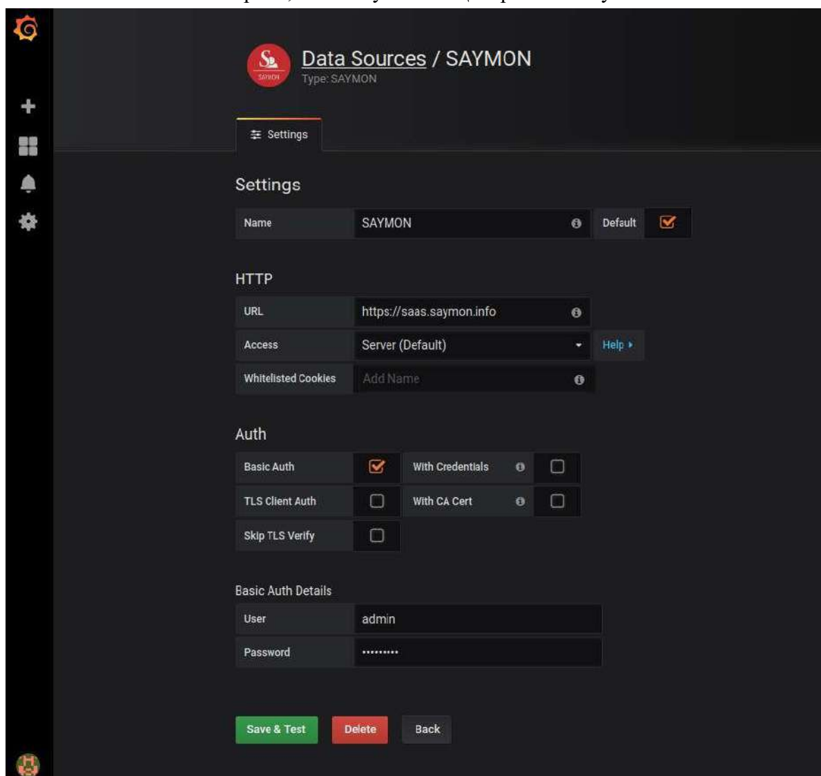
Рис. 3.5.2.3. Настройка источника данных в Grafana
