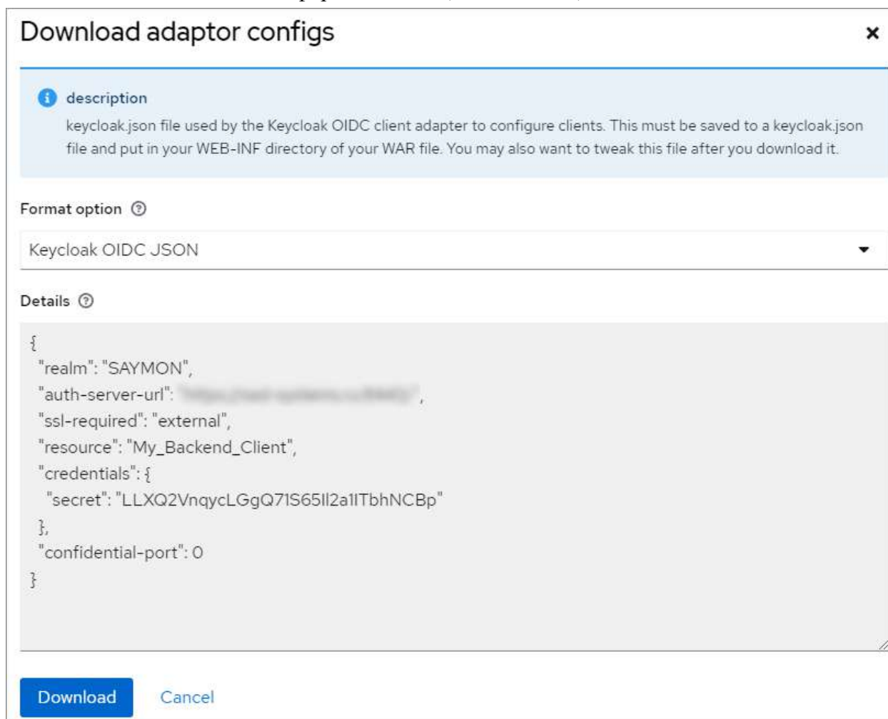
Рис. 3.5.3.1.9. Пример данных файла конфигурации Backend-клиента
