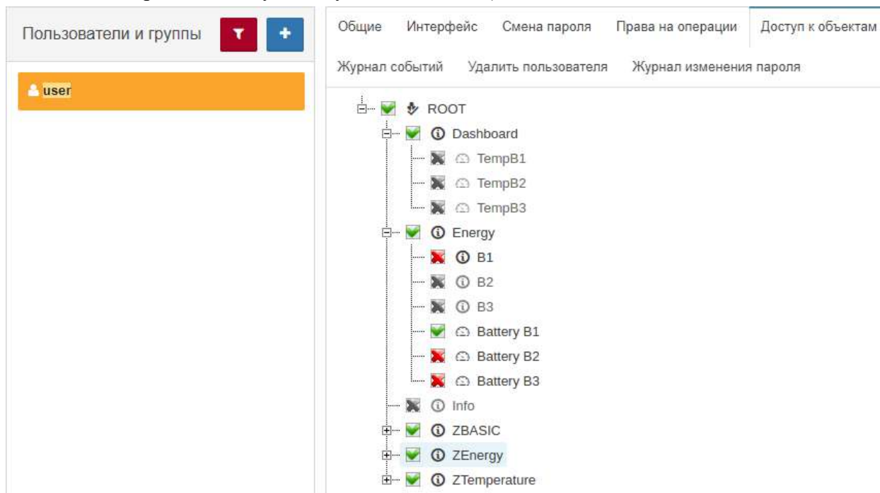
Рис. 3.7.7.1. Доступ к объектам
