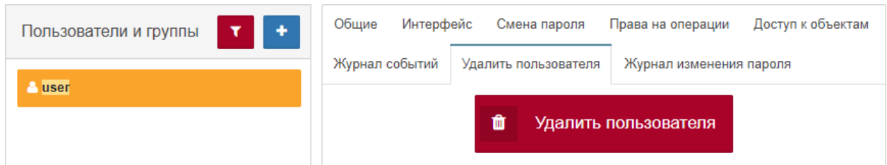
Рис. 3.7.9.1. Удаление пользователя
