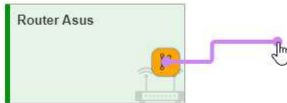
Рис. 3.8.5.1. Создание связи
